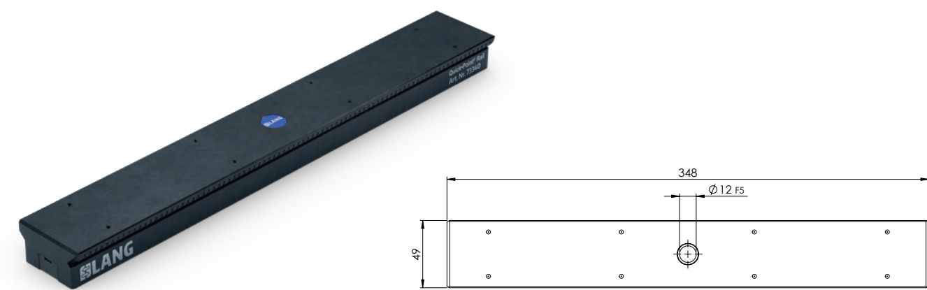
QUICK-POINT® RAIL, SPANNLEISTE OHNE BEFESTIGUNGSBOHRUNGEN
