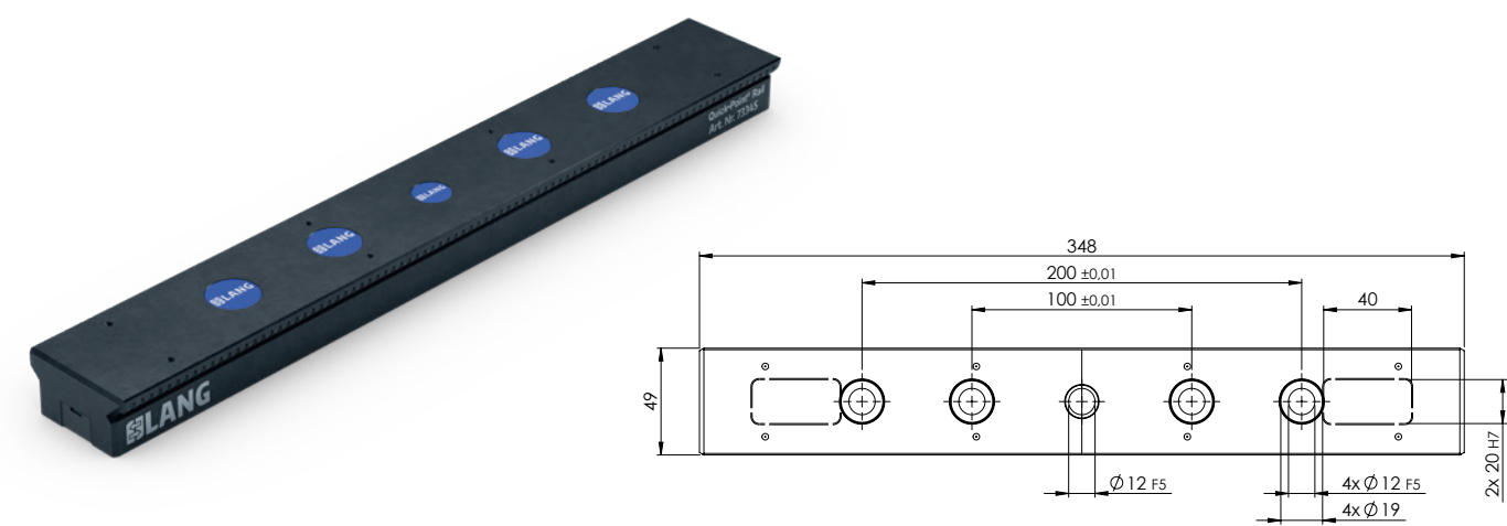
QUICK-POINT® RAIL, SPANNLEISTE MIT BEFESTIGUNGSBOHRUNGEN
