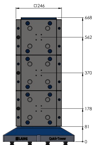
Quick-Tower hauteur 668 mm, avec 3 plaques Quick-Point® 75710 par face
