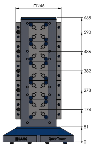
Quick·Tower hauteur 668 mm, avec 5 plaques Quick·Point® 75600 par face
