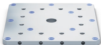
QUICK-TOWER FAUSSE PLAQUE, AVEC PERÇAGES CENTRAL DIAM. 50H7, AVEC PERÇAGES DE FIXATION
