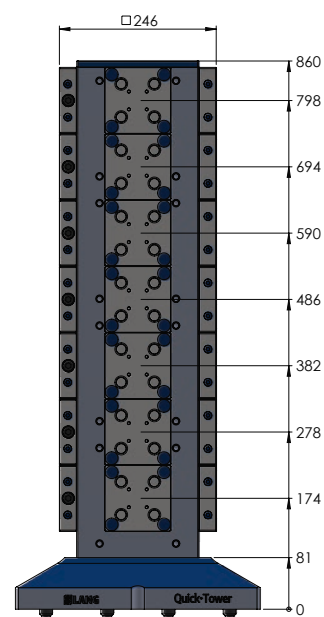
Quick·Tower hauteur 860 mm, avec 7 plaques Quick·Point® 75600 par face
