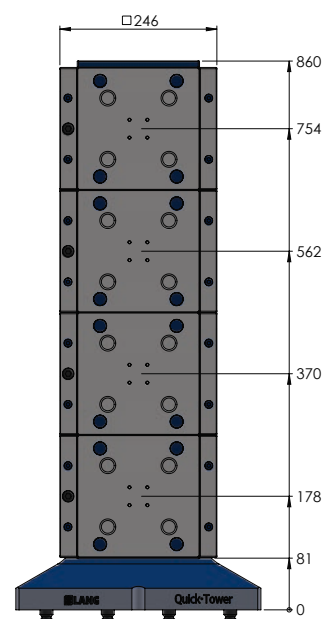
Quick-Tower hauteur 860 mm, avec 4 plaques Quick-Point® 75710 par face
